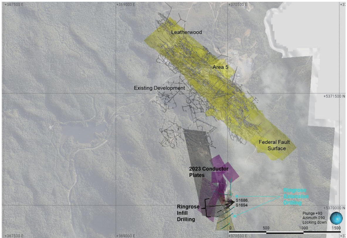
圖3.導體板位置規劃、礦化模型以及當前進行中的Ringrose填充及Ringrose延伸鑽探計劃。S1686及S1694是Ringrose填充計劃的一部分，並從同一鑽台位置進行接箍
