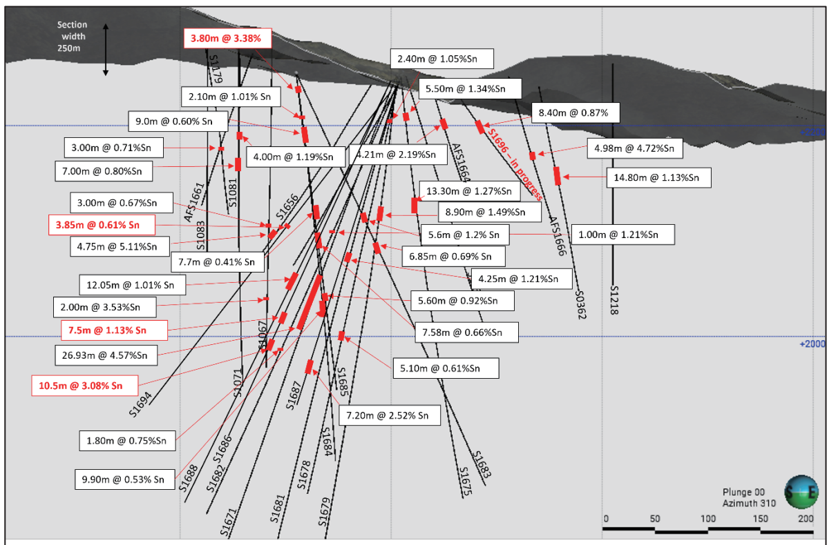
圖2：北向的剖面（250米寬）顯示新的（紅色文字）以及先前所報告及歷史的（黑色文字）錫交匯點。樣段顯示為井下寬度。
