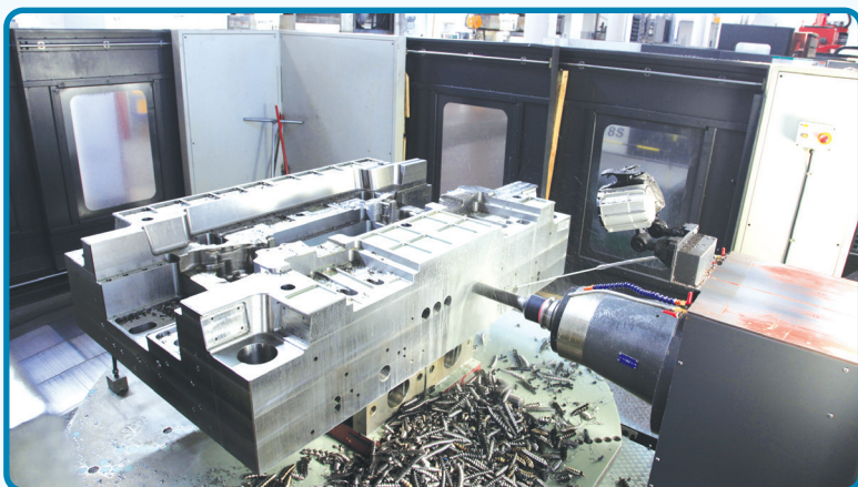
臥式加工中心正為一件大型非標模架進行切削形框及精孔
