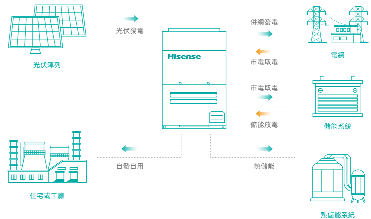
光儲直柔變頻中央空調系統
