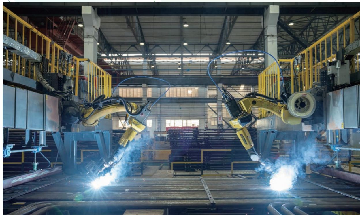
● 自主研发蛇形管附件焊接机器人系统、行业首台大型高压容器全自动激光封口焊上线，锅炉集箱高速数控钻成功实现“双机合璧”
