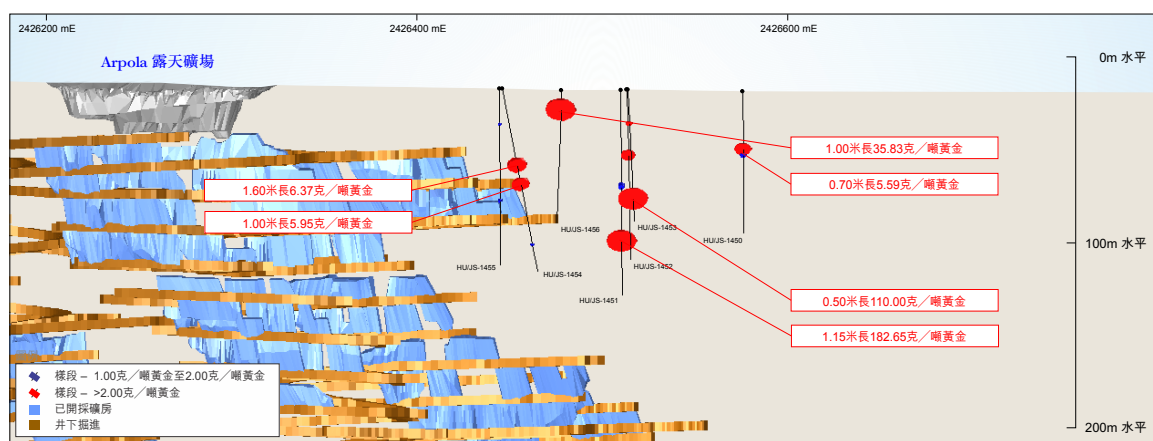
圖7－Jokisivu 勘探垂直剖面。向北視圖。
