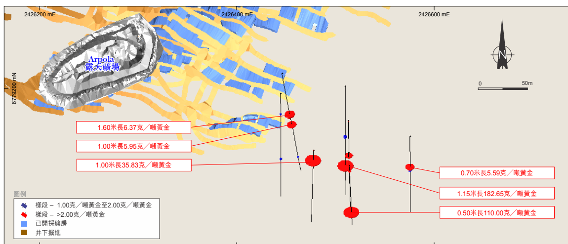
圖6－Jokisivu 勘探平面圖。
