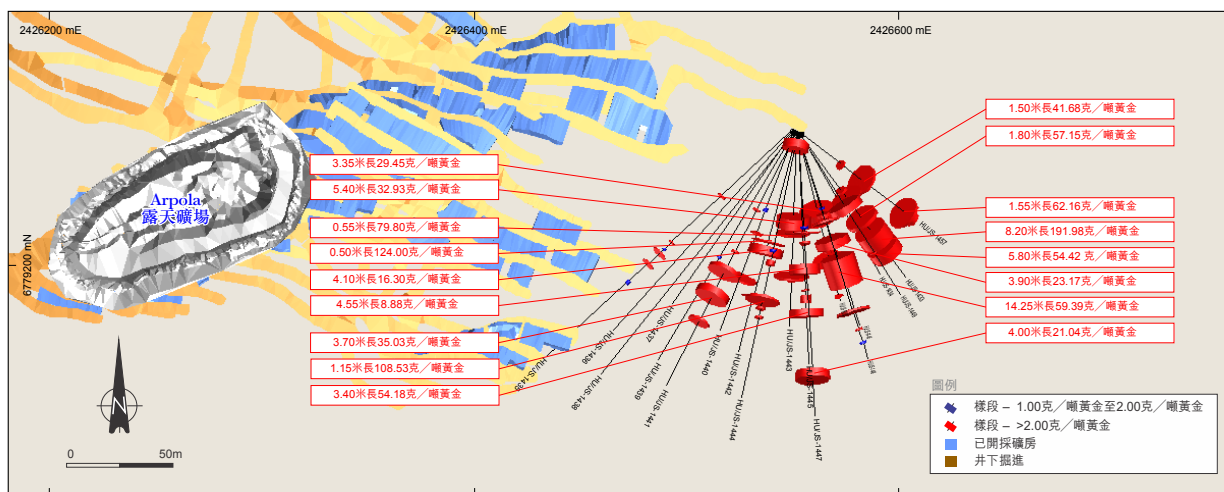
圖4—Arpola-3平面圖。
