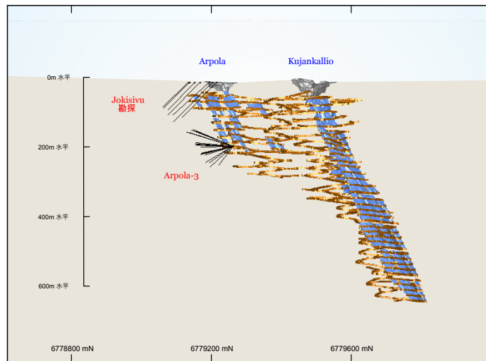
圖3－Jokisivu金礦顯示報告的鑽探位置。向西垂直視圖。
